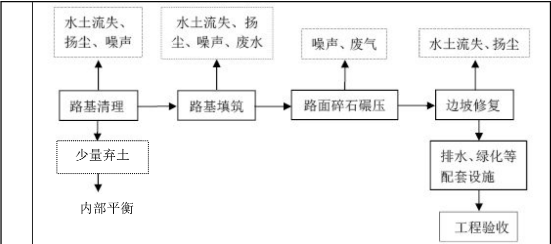
图 4-3 进场道路施工工艺及产污环节图
